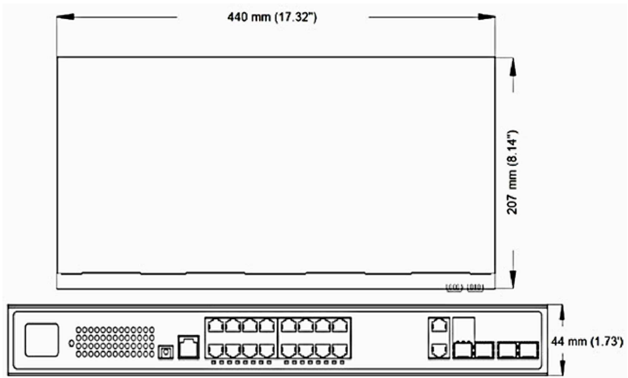
本体外観
